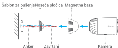
Slika 1 Montaža uz pomoć magnetne baze
