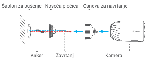
Slika 2 Montaža uz pomoć navojne baze
